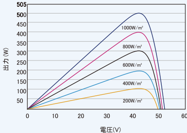
PVモジュール (500W) の P-V 曲線
